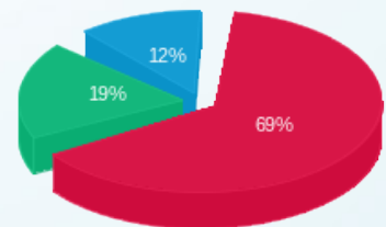
■ פסגה (Kwh 99,661.47) ■ גבע (Kwh 27,399.64) ■ שפל (Kwh 17,714.12)
