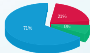
■ פסגה (22,838.71 Kwh) ■ גבע (8,521.79 Kwh) ■ שפל (76,814.27 Kwh)
