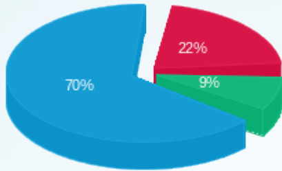
פסגה (Kwh 150,577.62) ■ גבע (Kwh 59,696.90) ■ שפל (Kwh 489,308.60) ■
