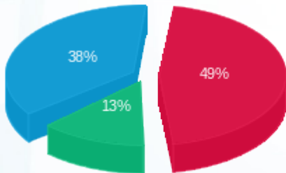
פסגה (Kwh 273,746.70) ■ גבע (Kwh 75,169.40) ■ שפל (Kwh 214,770.50) ■
