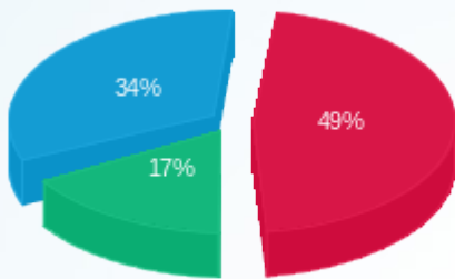
■ פסגה (38,990.20 Kwh) ■ גבע (13,241.95 Kwh) ■ שפל (26,984.75 Kwh)
