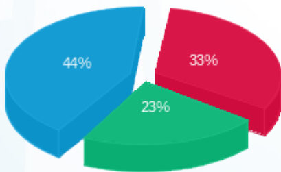
פסגה (Kwh 14,971.20) ■ גבע (Kwh 10,486.80) ■ שפל (Kwh 19,910.80) ■
