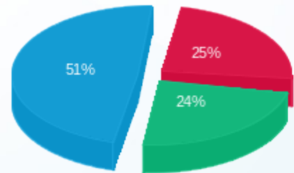
■ פסגה (Kwh 2,992.54) ■ גבע (Kwh 2,928.78) ■ שפל (Kwh 6,096.02)
