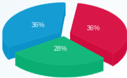
■ פסגה (259,116.20 Kwh) ■ גבע (201,331.20 Kwh) ■ שפל (255,739.90 Kwh)
