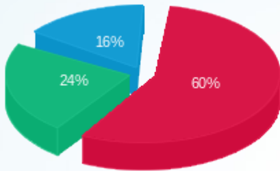
פסגה (Kwh 50,743.65) גבע (Kwh 20,163.26) שפל (Kwh 13,733.78)
