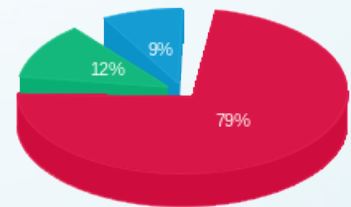
■ פסגה (36,901.48 Kwh) ■ גבע (5,658.03 Kwh) ■ שפל (4,106.95 Kwh)
