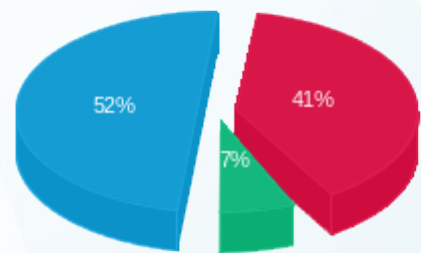
■ פסגה (567.93 Kwh) ■ גבע (90.56 Kwh) ■ שפל (715.39 Kwh)
