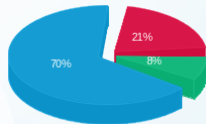
■ פסגה (Kwh 126,425.70) ■ גבע (Kwh 48,865.54) ■ שפל (Kwh 418,049.39)
