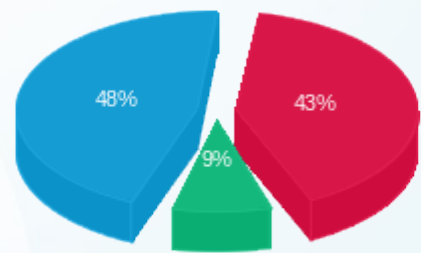
פסגה (Kwh 10,344.03) ■ גבע (Kwh 2,092.12) ■ שפל (Kwh 11,442.57) ■
