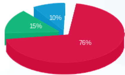
■ פסגה (238.24 kWh) ■ גבע (45.68 kWh) ■ שפל (30.54 kWh)
