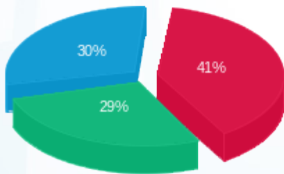
■ פסגה (Kwh 93,944.15) ■ גבע (Kwh 65,577.15) ■ שפל (Kwh 68,052.47)
