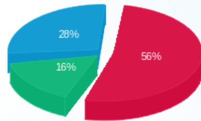
■ פסגה (36,009.68 Kwh) ■ גבע (10,566.53 Kwh) ■ שפל (18,120.82 Kwh)
