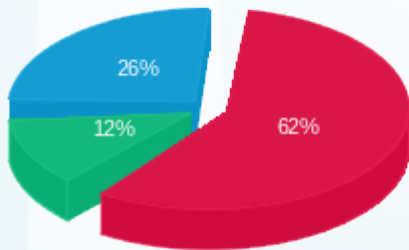
■ פסגה (Kwh 89,917.78) 62% ■ גבע (Kwh 17,267.50) 12% ■ שפל (Kwh 37,798.12) 26%
