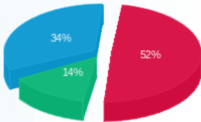
■ פסגה (Kwh 205,588.67) ■ גבע (Kwh 56,666.60) ■ שפל (Kwh 134,944.90)
