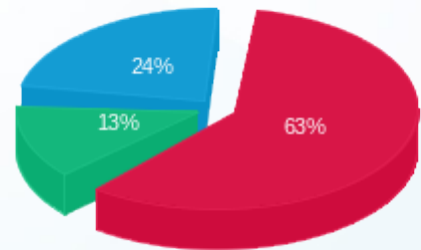
■ פסגה (7,089.98 Kwh) ■ גבע (1,446.84 Kwh) ■ שפל (2,645.94 Kwh)
