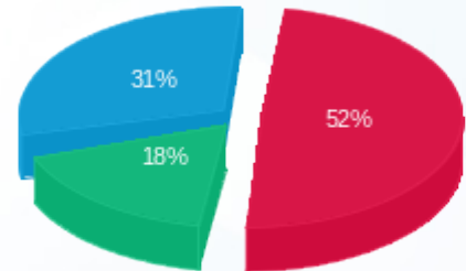
■ פסגה (Kwh 14,289.05) ■ גבע (Kwh 4,936.11) ■ שפל (Kwh 8,499.50)
