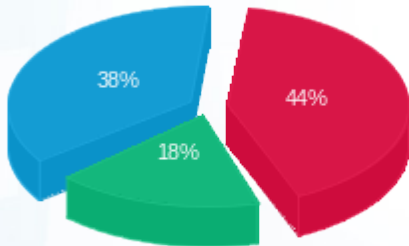
■ פסגה (Kwh 31,411.40) ■ גבע (Kwh 13,086.20) ■ שפל (Kwh 27,242.00)
