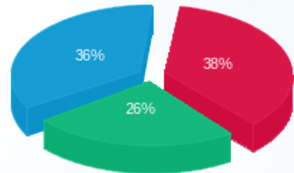
■ פסגה (47,943.10 Kwh) ■ גבע (32,939.30 Kwh) ■ שפל (46,273.10 Kwh)
