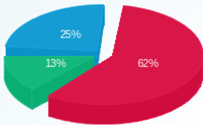
■ פסגה (10,679.40 Kwh) ■ גבע (2,188.55 Kwh) ■ שפל (4,242.90 Kwh)
