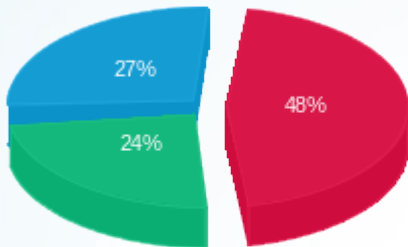
פסגה (Kwh 145,713.77) ■ גבע (Kwh 73,345.89) ■ שפל (Kwh 82,118.86) ■
