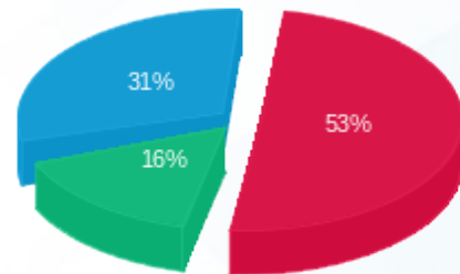
■ פסגה (96,396.00 Kwh) ■ גבע (29,356.00 Kwh) ■ שפל (57,132.00 Kwh)
