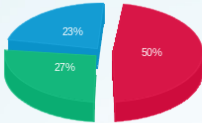
פסגה (Kwh 171,238.35) ■ גבע (Kwh 92,348.01) ■ שפל (Kwh 79,317.55) ■
