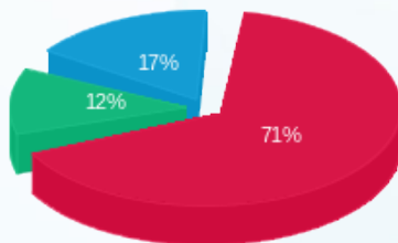
■ פסגה (168,810.00 Kwh) ■ גבע (28,951.60 Kwh) ■ שפל (39,666.80 Kwh)
