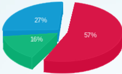
■ פסגה (Kwh 80,785.58) ■ גבע (Kwh 21,810.50) ■ שפל (Kwh 37,993.15)
