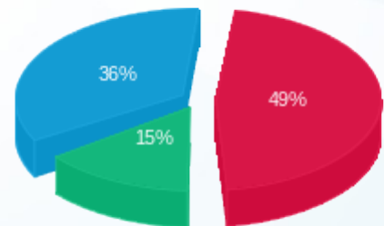
■ פסגה (Kwh 127,512.04) ■ גבע (Kwh 38,269.26) ■ שפל (Kwh 93,392.55)
