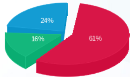
■ פסגה (38,210.08 Kwh) ■ גבע (9,726.60 Kwh) ■ שפל (14,730.03 Kwh)
