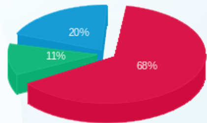
פסגה (Kwh 15,511.94) 68% גבע (Kwh 2,506.05) 11% שפל (Kwh 4,564.28) 20%
