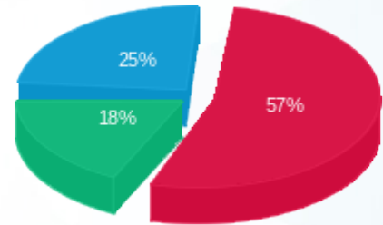
■ פסגה (Kwh 222,340.53) ■ גבע (Kwh 71,795.04) ■ שפל (Kwh 98,022.14)
