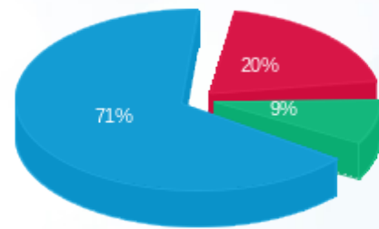
■ פסגה (Kwh 42,274.26) ■ גבע (Kwh 18,037.45) ■ שפל (Kwh 146,113.98)
