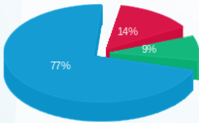
■ פסגה (Kwh 202,291.49) ■ גבע (Kwh 132,313.34) ■ שפל (Kwh 1,124,815.06)
