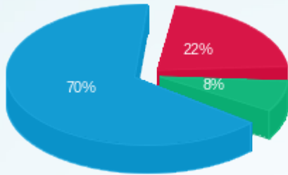
■ פסגה (Kwh 39,496.00) ■ גבע (Kwh 13,990.40) ■ שפל (Kwh 125,423.60)
