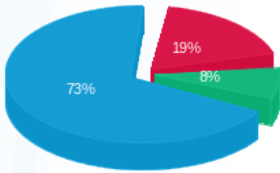
■ פסגה (910.40 Kwh) ■ גבע (397.80 Kwh) ■ שפל (3,545.60 Kwh)
