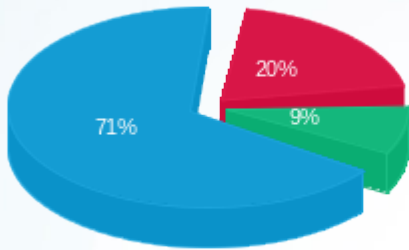
■ פסגה (12,277.60 Kwh) ■ גבע (5,143.30 Kwh) ■ שפל (42,849.90 Kwh)
