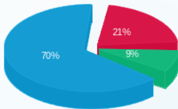
■ פסגה (Kwh 33,224.55) ■ גבע (Kwh 13,889.90) ■ שפל (Kwh 108,081.30)
