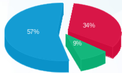
■ פסגה (5,230.33 Kwh) ■ גבע (1,342.09 Kwh) ■ שפל (8,823.44 Kwh)
