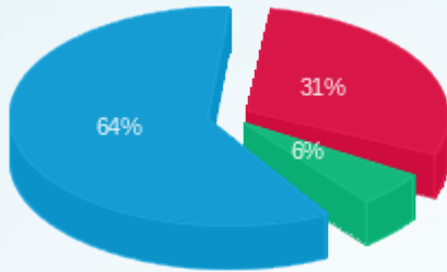
פסגה (Kwh 158,422.95) ■ גבע (Kwh 29,355.83) ■ שפל (Kwh 329,464.66) ■
