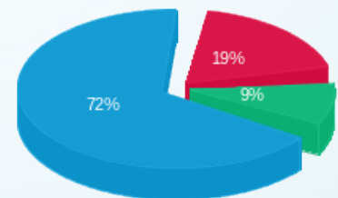
■ פסגה (Kwh 44,776.60) ■ גבע (Kwh 21,589.40) ■ שפל (Kwh 166,536.00)
