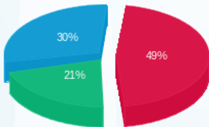
■ פסגה (Kwh 220,198.90) ■ גבע (Kwh 94,896.99) ■ שפל (Kwh 134,313.51)
