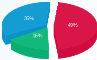
פסגה (Kwh 44,208.72) ■ גבע (Kwh 14,808.54) ■ שפל (Kwh 31,876.30) ■
