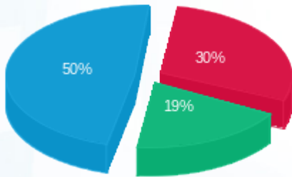
■ פסגה (Kwh 11,523.66) ■ גבע (Kwh 7,353.91) ■ שפל (Kwh 19,079.24)
