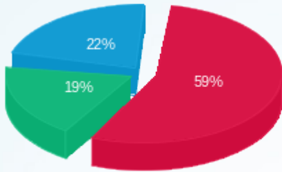
■ פסגה (Kwh 421,802.16) ■ גבע (Kwh 134,494.38) ■ שפל (Kwh 160,645.98)
