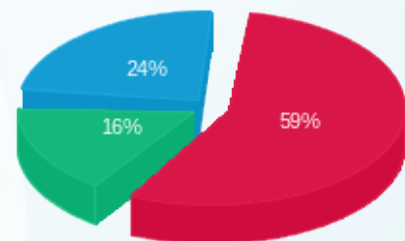
■ פסגה (22,955.50 Kwh) ■ גבע (6,240.20 Kwh) ■ שפל (9,396.84 Kwh)
