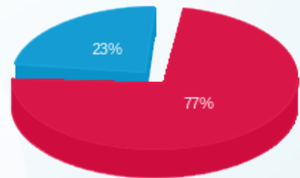
פסגה (Kwh 393,305.10) 77% גבע (Kwh 0.00) 0% שפל (Kwh 120,146.29) 23%
