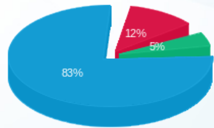
■ פסגה (Kwh 49,245.26) ■ גבע (Kwh 19,796.50) ■ שפל (Kwh 341,344.21)
