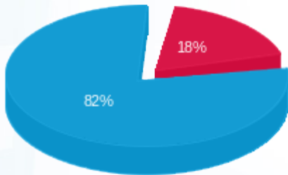
■ פסגה (11,959.90 Kwh) ■ גבע (0.00 Kwh) ■ שפל (55,260.22 Kwh)
