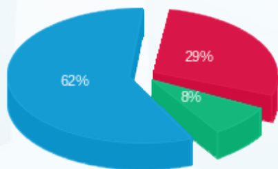
■ פסגה (Kwh 160,068.33) ■ גבע (Kwh 45,989.61) ■ שפל (Kwh 338,111.83)
