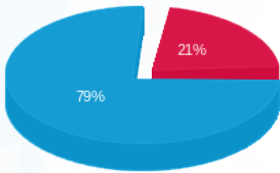
■ פסגה (64,418.70 Kwh) ■ גבע (0.00 Kwh) ■ שפל (241,981.25 Kwh)
